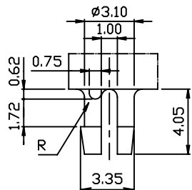
DETAIL Y
